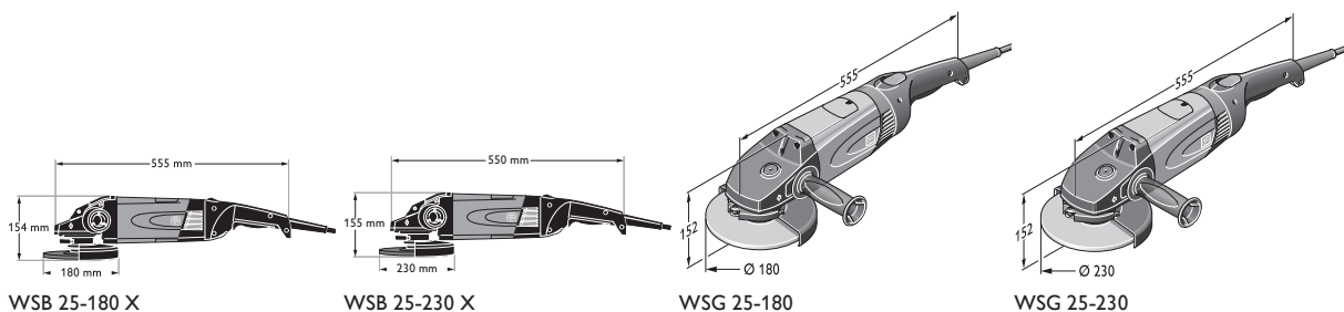
WSB 25-180 X
