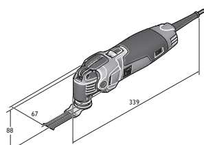
FMM 350 QSL
