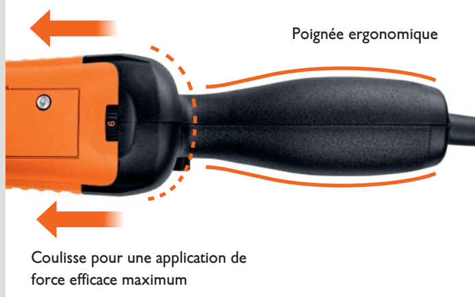
Meuleuse droite à poignée FEIN ERGOGRIP GSZ 11-320 PERL
