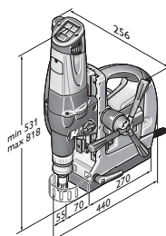
КБМ 80 auto
