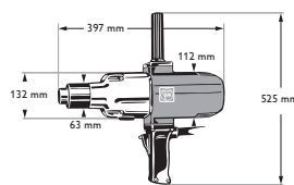
DDSk 672-1
