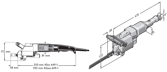
AStx 649-1 AStxe 649-1
