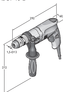
ВОР 10-2
