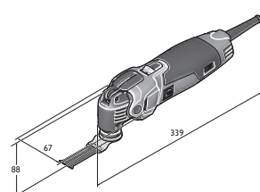
AFMM 350 QSL
