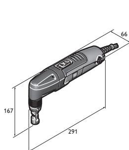
BLK 2.0 E
