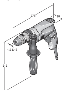
ВОР 10
