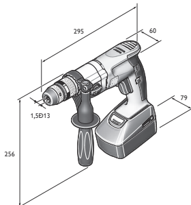
АВОР 13-2
