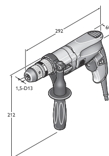
ВОР 13-2
