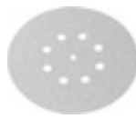
brusné listy děrovaný, Ø 150 mm, s rychlým upevněním suchým zipem Oblast použití: Kov, neopracované karosérie motorových vozidel, spájené spoje, svary, umělá hmota tvrděná skelným vláknem. Kvalita: Vysoce výkonná brusná látka, spojená plně syntetickou pryskyřicí, korund. Vlastnost: velmi stabilní, vysoký úběrový výkon.
