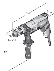
BOP 13-2
