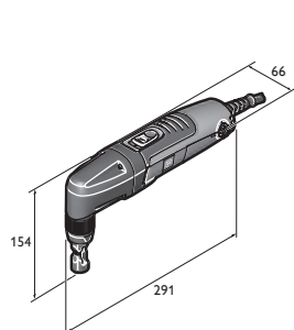
BLK 1.6 E
