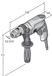
BOP 6
