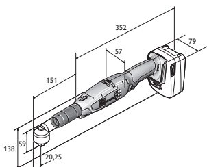
ASW 18-60 PC
