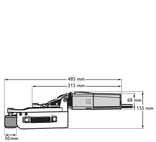
RS 12-70 E
