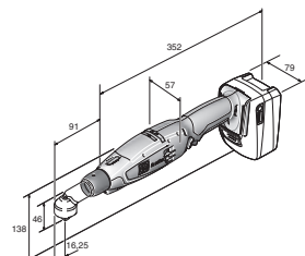
ASW 18-18 PC
