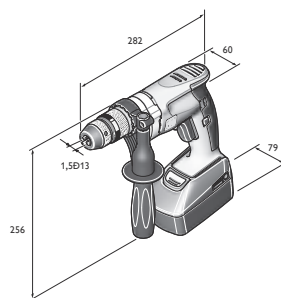
ABOP 10
