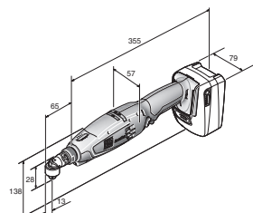
ASW 18-6
