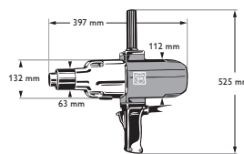
DDSk 672-1
