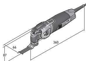
AFSC 500 QSL
