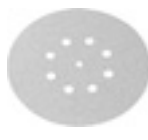
Arkusze ścierne z perforacją, Ø 150 mm, z szybkim mocowaniem na rzep Zakres zastosowań: drewno, farba, lakiery samochodowe, masa szpachlowa, tworzywa sztuczne i TWS. Jakość: związane żywicą syntetyczną, korund. Właściwość: znacznie zmniejszone zatykanie się, elastyczność.
